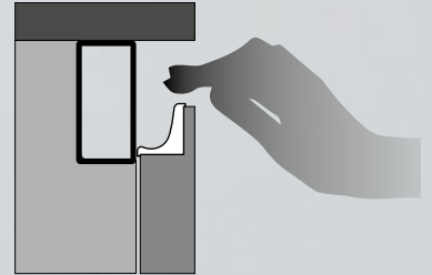
GORGE "DROITE" AVEC POIGNÉE ENCASTRÉE Ranura "Recta" con tirador acanalado
