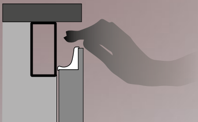
PRISE DE MAIN "FRAME" Tirador acanalado "Frame"
